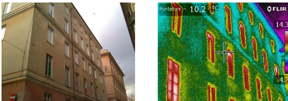
Figura.2 – Rilievo termografico del prospetto esterno - Via Tollot
