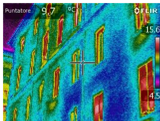
Figura 3 – Rilievo termografico dei serramenti esterni – Facciata posteriore – Via Tollot
